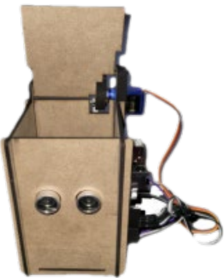
아두이노 자동감지 휴지통
